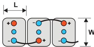
TYPE 2ETG 100 to 600
